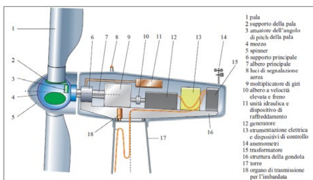
Struttura tipica di una turbina eolica
